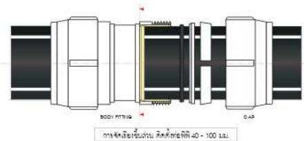
การใช้งานเชื่อมระบบ ดึงที่ท่อขนาด 40 - 100 มม.
