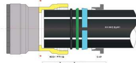
การใช้งานเชื่อมระบบ ดึงที่ท่อขนาด 100 - 250 มม.
